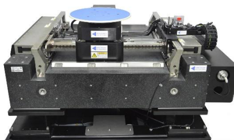
Akribis linjära servomotorer och linjära steg
